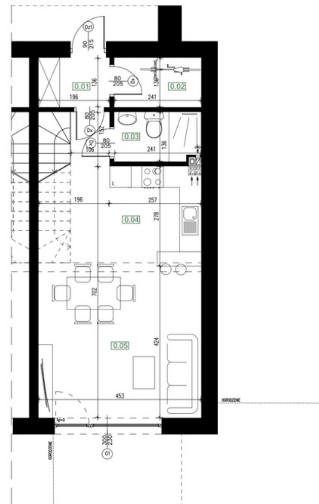
RZUT PARTERU
